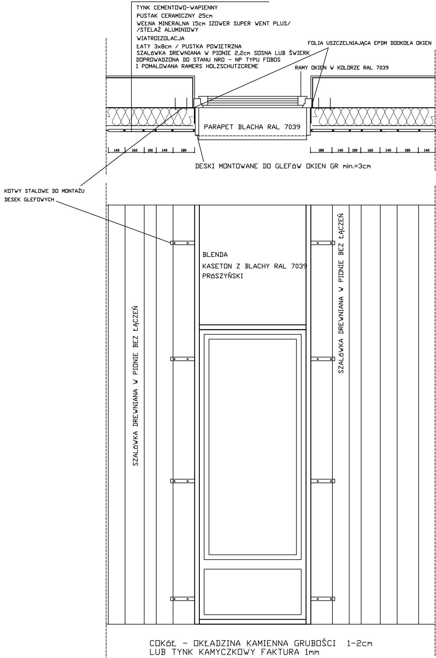
DETAL OKŁADZINY ŚCIANY ZEWNĘTRZNEJ WRAZ Z OKNEM SKALA 1:20
